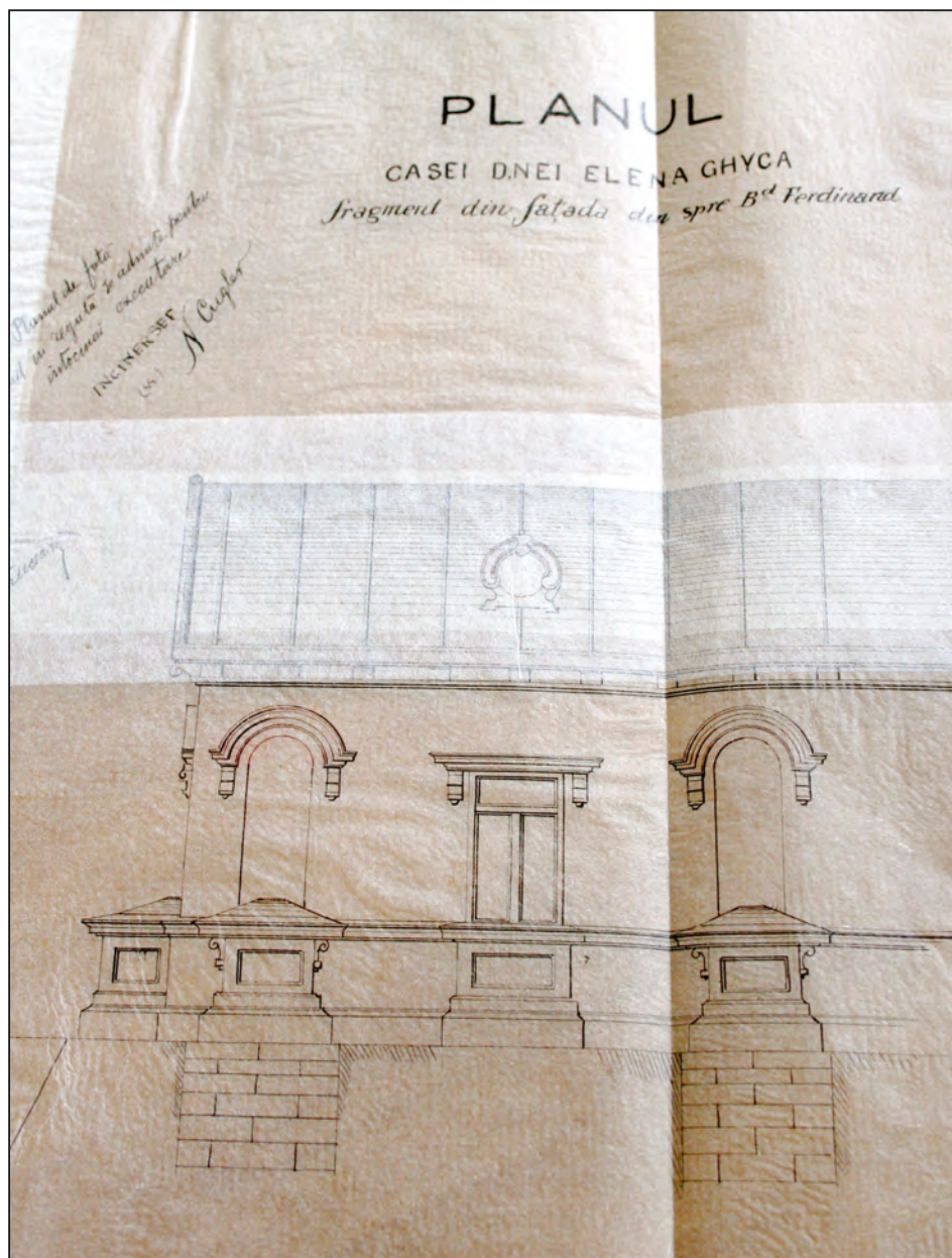
Fig. 3 - Planul casei Ghica detaliu
